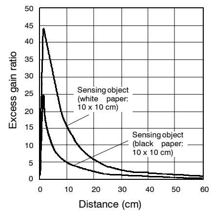
E3F2-DS30□4 E3F2-DS30□4-P1
