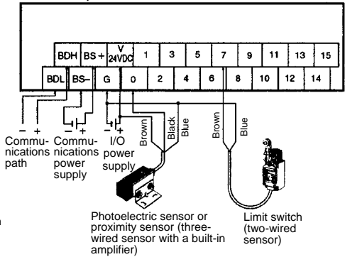
SRT1-ID16, SRT2-ID16
