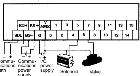
SRT1-OD16, SRT2-OD16
