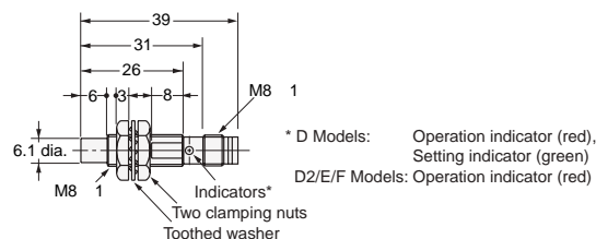
Diagram 29 E2E-X4MD□-M3G/E2E-X2ME□-M3/X2MF□-M3
